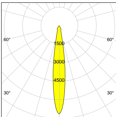
I-max : 7154 cd/klm *
