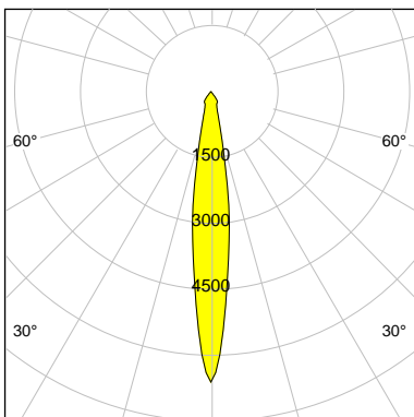
I-max : 6603 cd/klm *
