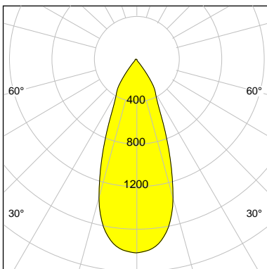
I-max : 1821 cd/klm *
